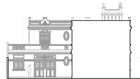
Elevation 04
